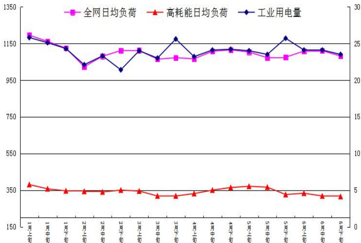
用电负荷（万千瓦） 全区工业用电量及用电负荷变化趋势图 用电量（亿千瓦时）
