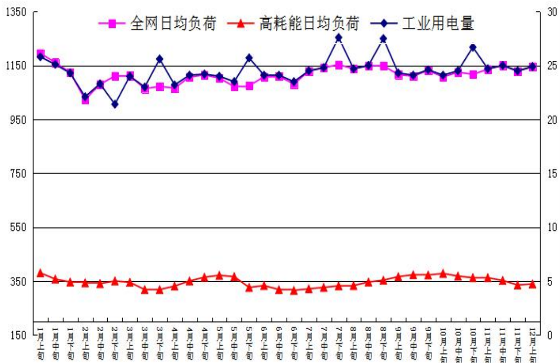
用电负荷（万千瓦） 全区工业用电量及用电负荷变化趋势图 用电量（亿千瓦时）
