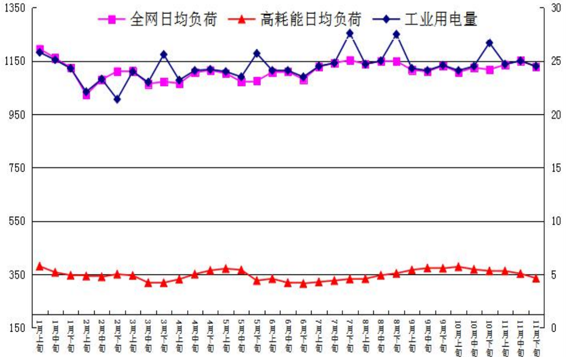
全区工业用电量及用电负荷变化趋势图
