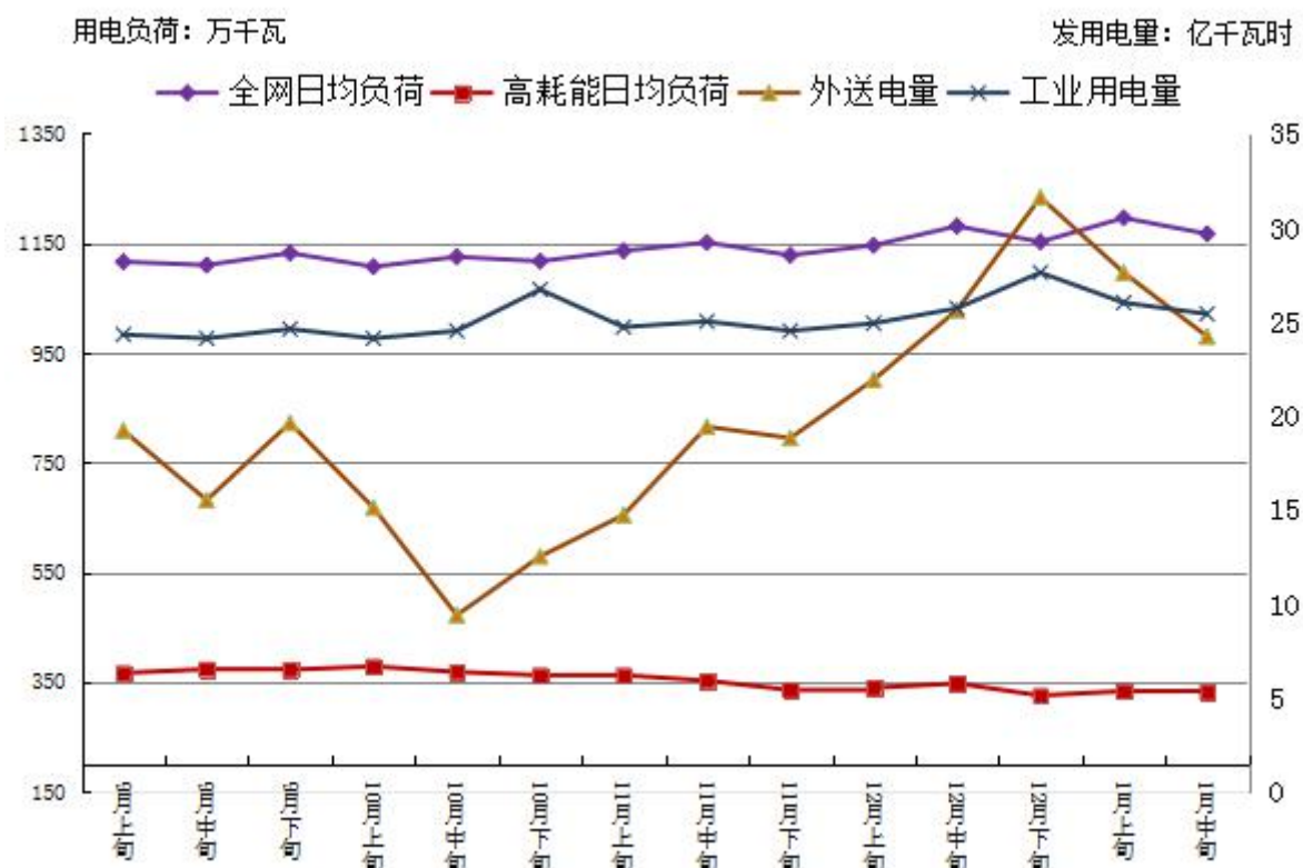
全区工业用电、外送电量及用电负荷变化趋势图
