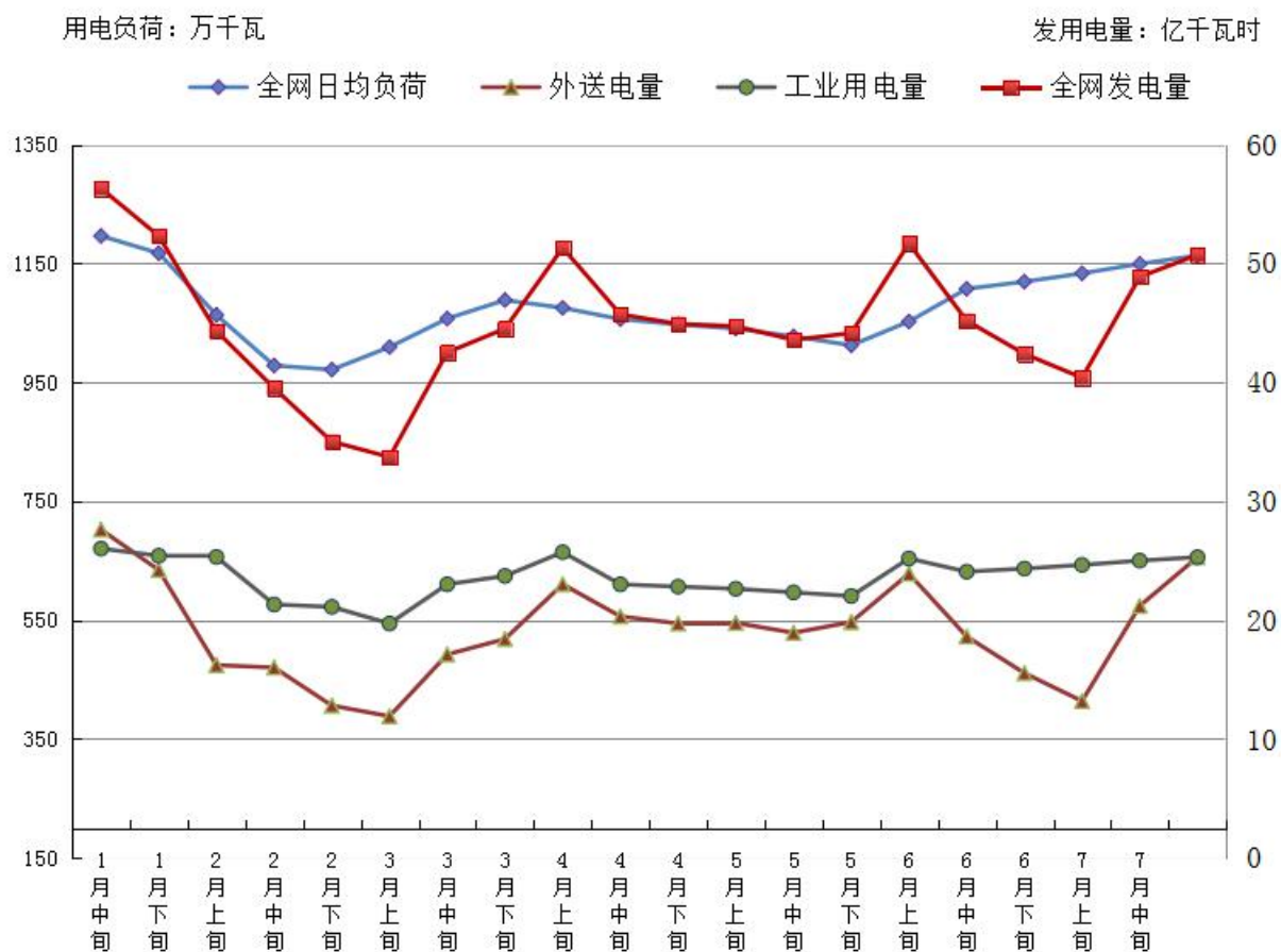
全区工业用电、外送电量及用电负荷变化趋势图
